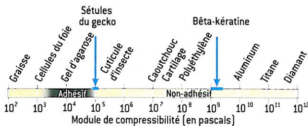
7. Le module de Young décrit la rigidité d'une substance. Bien que le module de compressibilité (une quantité associée au module de Young) de la bêta-kératine massive soit d'environ deux milliards de pascals, le module des sétules est plus de 10 000 fois inférieur; au-dessous, les substances sont adhésives (et stables), tandis qu'au-dessus, elles ne sont pas adhésives. Les sétules du gecko sont à la limite des deux domaines. Cette valeur autorise une adhérence forte et rapide tout en évitant un attachement spontané ou inapproprié.
