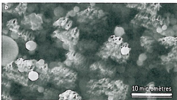
6. Les pattes des geckos sont autonettoyantes. Quand elles sont salies par des billes de cinq micromètres de diamètre [a, la flèche rouge indique une bille adhérant à plusieurs spatules], la plupart des débris disparaissent (b) après quatre pas sur du verre propre.
