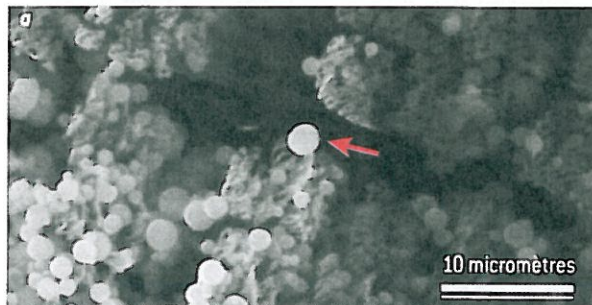
5. La forte adhérence entre la surface hydrophobe des doigts du gecko tokay et la surface hydrophobe très lisse de l'arséniure de gallium prouve que les forces de Van der Waals suffisent à assurer l'adhérence du gecko.
